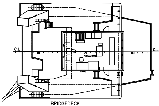
BRIDGEDECK
